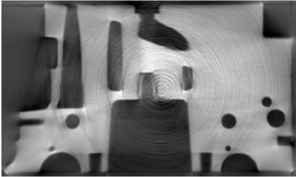
2. ábra Gyűrű műtermékek egy VW hengerfej186 CT felvételen
